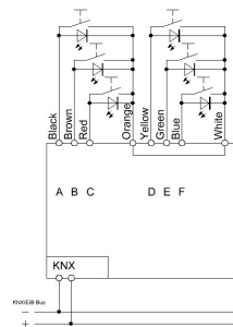
Anschlussbeispiel BE-06001.02 - Circuit diagram BE-06000.01
